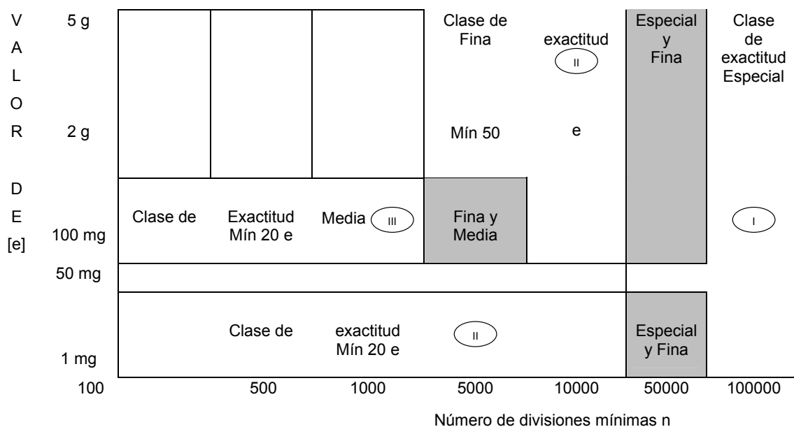
Figura 3: Clasificación de los instrumentos para pesar
