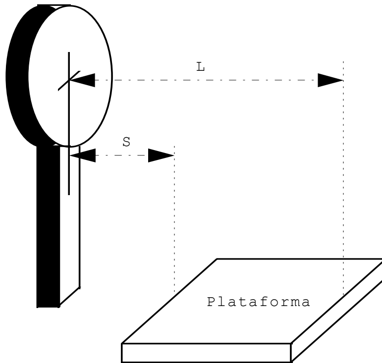
FIGURA 1.- La distancia mínima de lectura es S ; si S < 0,8 m, la distancia mínima de lectura es L .
